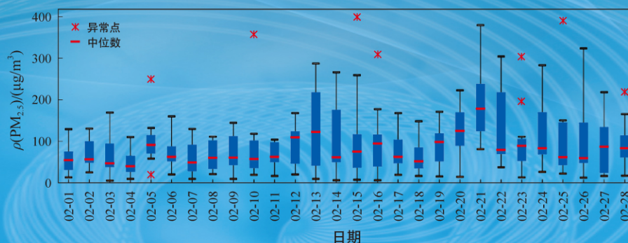
2006-2016年冬奥会同期北京奥体中心 \rho(\text{PM}_{2.5}) 日均值变化
